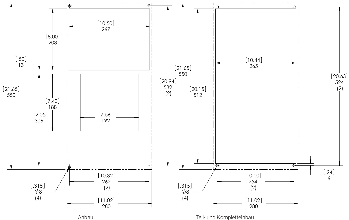
500 W AUSSCHNITTZEICHNUNG Gestrichelte Linien = Kühlgerät
